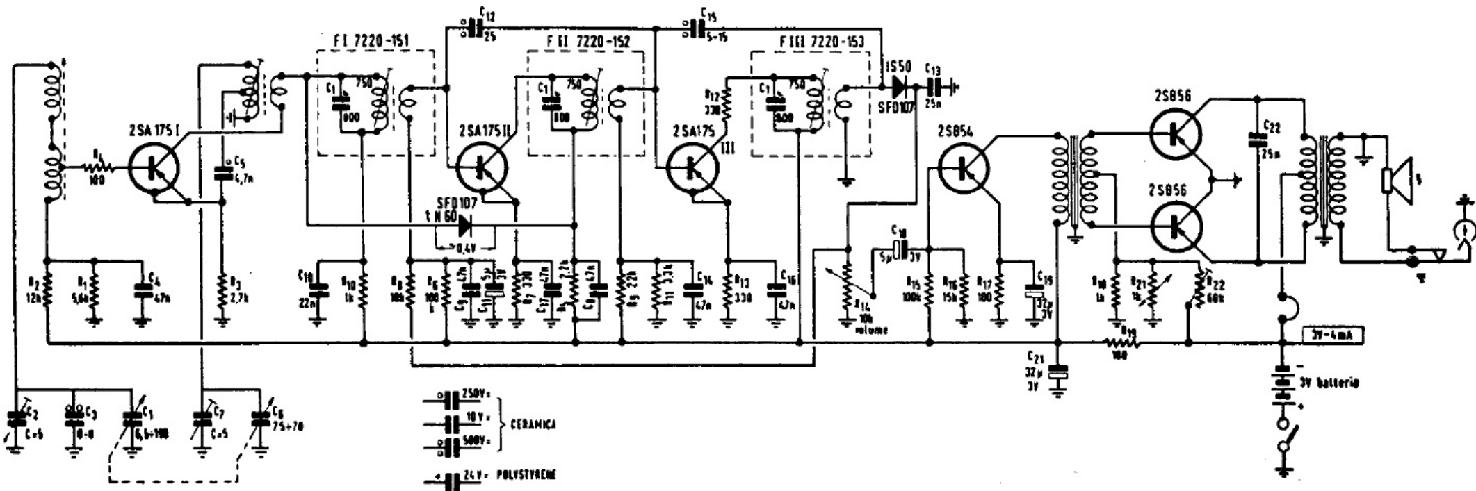
Schema elettrico del radioricevitore transistorizzato CRUNDIG mod. Solo-Boy 201
